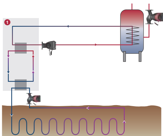
Fig. 10 Sistema de bombas de calor geotérmicas en un edificio comercial
