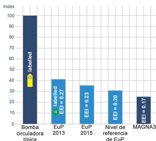
Fig. 55 Índice de consumo energético
