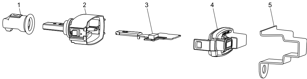
Fig. 37 Sensor
