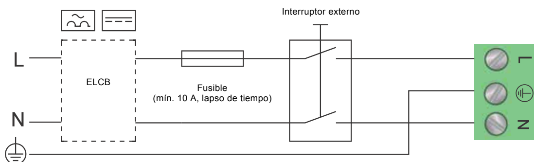
Fig. 39 Ejemplo de conexión habitual, 1 x 230 V \pm 10 %, 50/60 Hz
