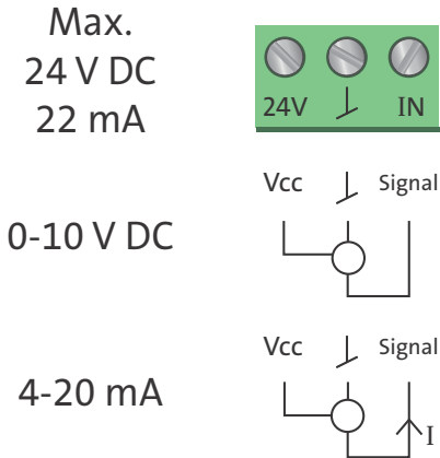
Fig. 44 Cableado, entrada analógica
